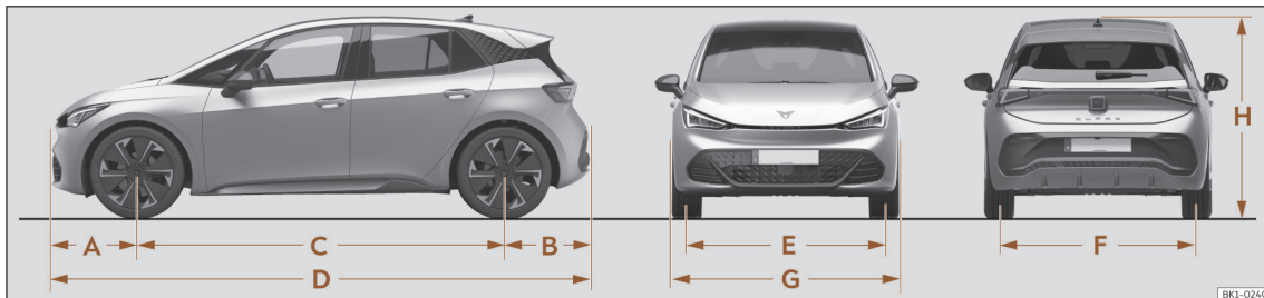
Afb. 204 Afmetingen
