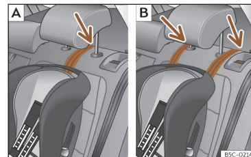
Afb. 41 Stoelen achterin: afstelling en montage volgens de Top Tether-gordel.
