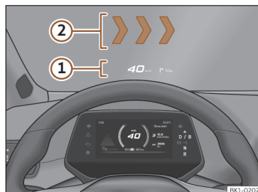
Afb. 4 In het gezichtsveld van de bestuurder: Proximity HUD ① en AR HUD ②.
