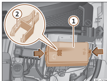
Afb. 181 In de voorruimte: deksel van de zekeringenhouder.
