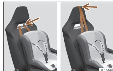
Afb. 42 Bijrijdersstoel: afstelling en montage volgens de Top Tether-gordel.
