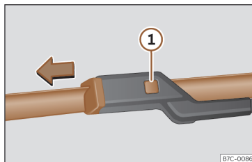
Afb. 173 Ruitenwischerbladen voorruit vervangen.
