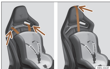
Afb. 43 Bijrijdersstoel: afstelling en montage volgens de Top Tether-gordel.
