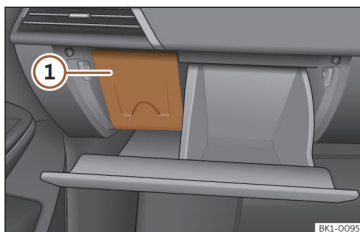
Afb. 180 Wagens met stuur rechts: afdekking van de zekeringhouder van het dashboard aan bestuurderszijde.
