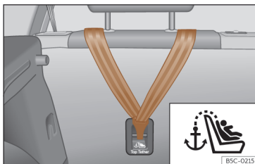
Afb. 39 Achterzijde van de achterstoelen: verankerung voor de Top Tether-riem.
