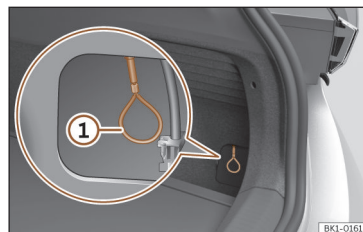
Afb. 62 Achter de afdekking: noodontgrendeling van de laadsteker.
