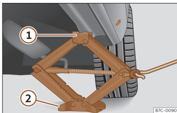
Afb. 197 Langsligger: plaatsing van de wagenkrik.
