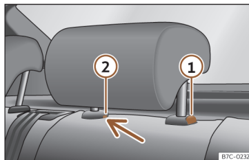
Afb. 102 Hoofdsteun achterin: verwijderen.
