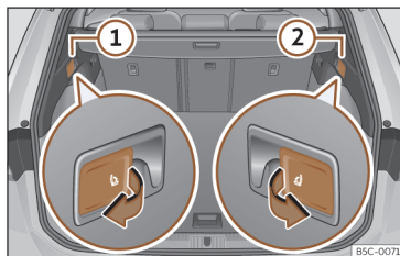
Afb. 106 In de bagageruimte: hendels voor ontgrendeling van de achterste rugleuning.
