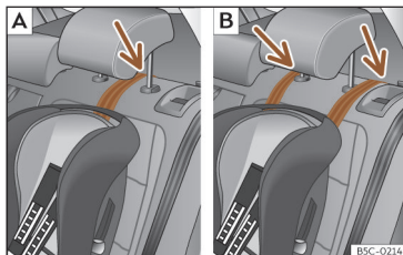
Afb. 45 Stoeien achterin: afstelling en montage volgens de Top Tether-gordel.
