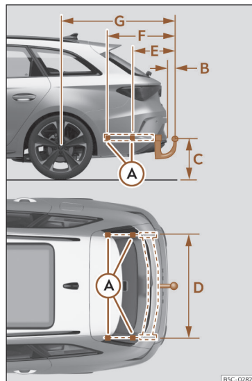
Afb. 212 Maten en bevestigingspunten voor het achteraf inbouwen van een trekhaak.
