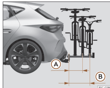
Afb. 211 Schematische voorstelling van de maximale overhang van de lading in een fietsendrager voor twee of drie fietsen.
