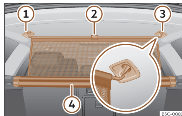
Afb. 195 In de bagageruimte: scheidingsnet inhaken.
