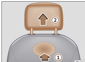
Afb. 101 Hoofdsteun voorin: demontage.
