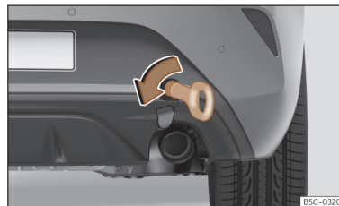
Afb. 228 Leon. Aan de rechterzijde van de achterbumper: vastgeschroefd sleepoog.
