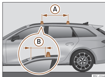
Afb. 206 Bevestigingspunten van de dwarsdragers voor het dakdragersysteem (Leon Sportstourer).
