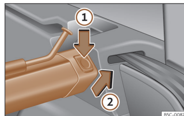
Afb. 196 In de bagageruimte: scheidingsnet uitbouwen.
