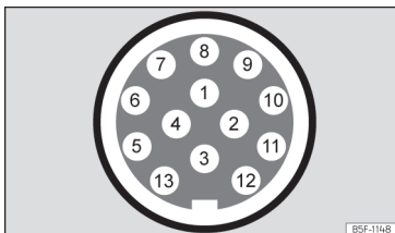
Afb. 208 Schematische weergave: toewijzing van de pinnen van het stopcontact voor de aanhangwagen.
