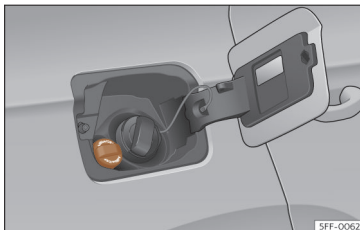
Afb. 216 Dop van de vulopening van de AdBlue®-tank.
