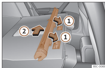
Afb. 197 Scheidingsnet op de rugleuningen van de achterbank inbouwen.
