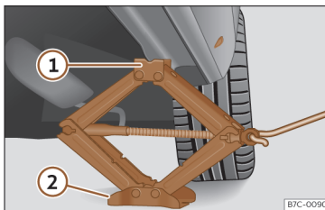
Afb. 256 Langsligger: plaatsing van de wagenkrik.
