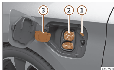
Afb. 62 Achter de laadklep van de accu, rechtsachter: laadcontactdoos.
