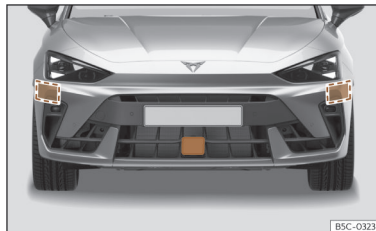
Afb. 131 In de voorbumper: radarsensoren vooraan en aan de zijkanten.
