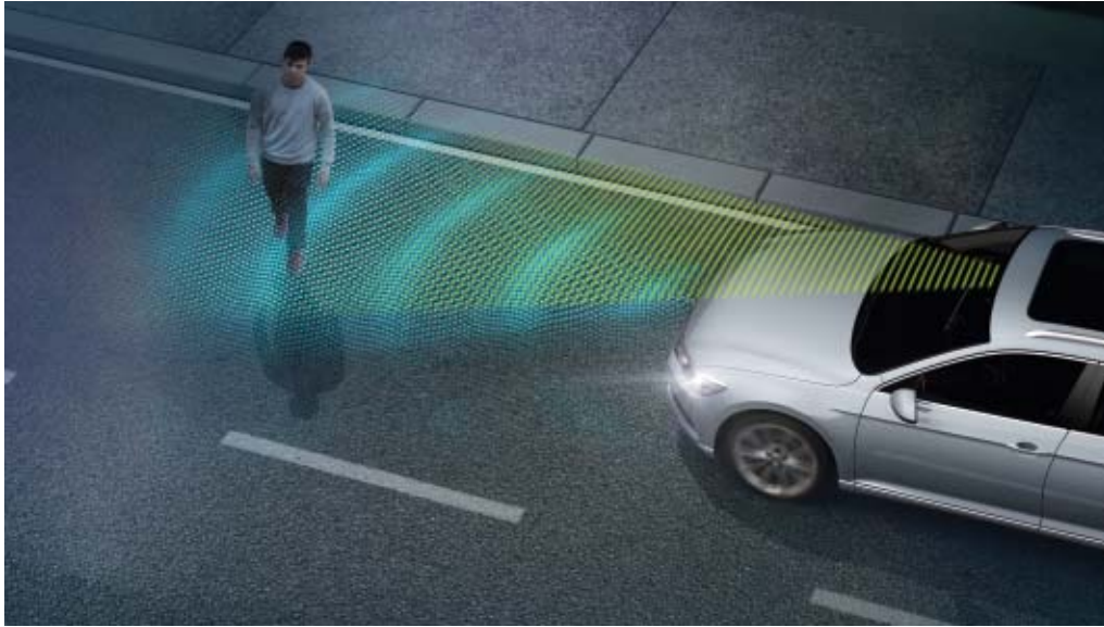
Voetgangersherkenning
